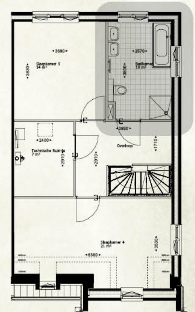
Extra badkamer 2e verdieping
