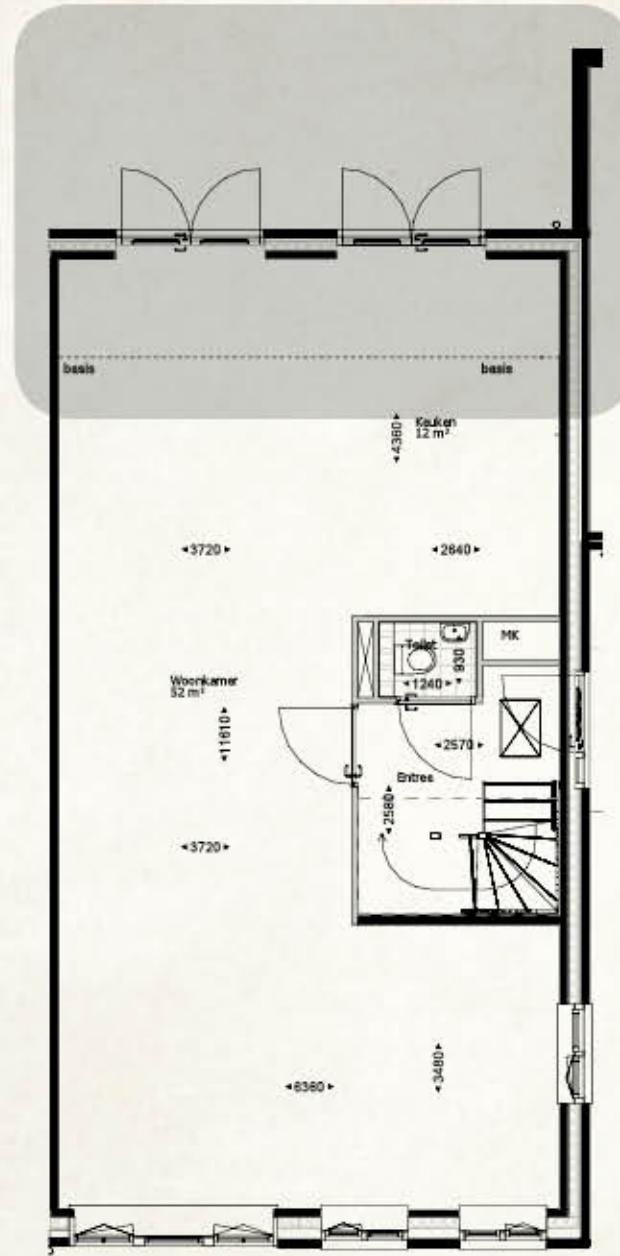
Uitbouw 1.2m Plattegrond op basis van type D1
