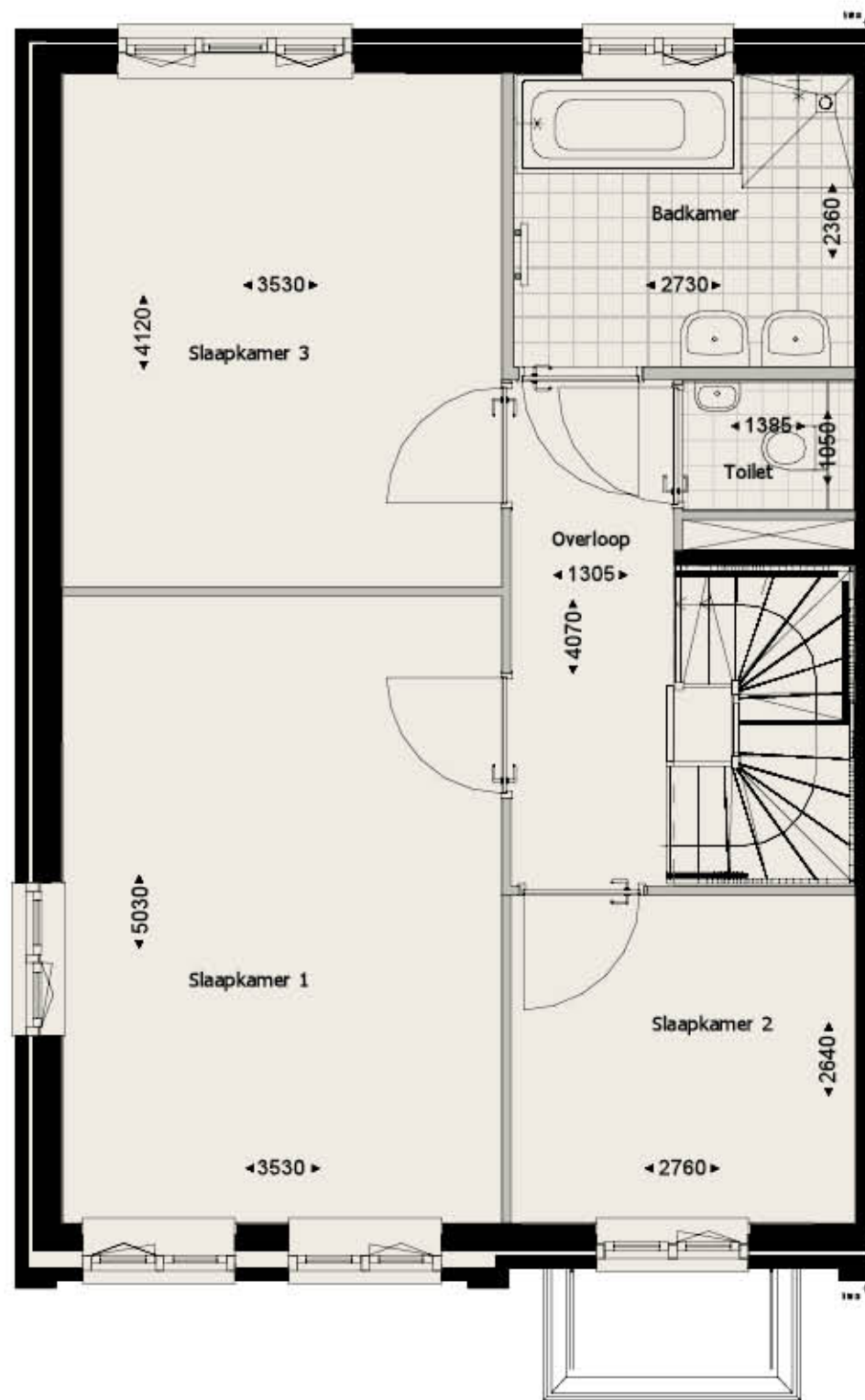
Eerste verdieping bouwnummer 30 en 33 (zoals afgebeeld) en 31 en 27 (gespiegeld)
