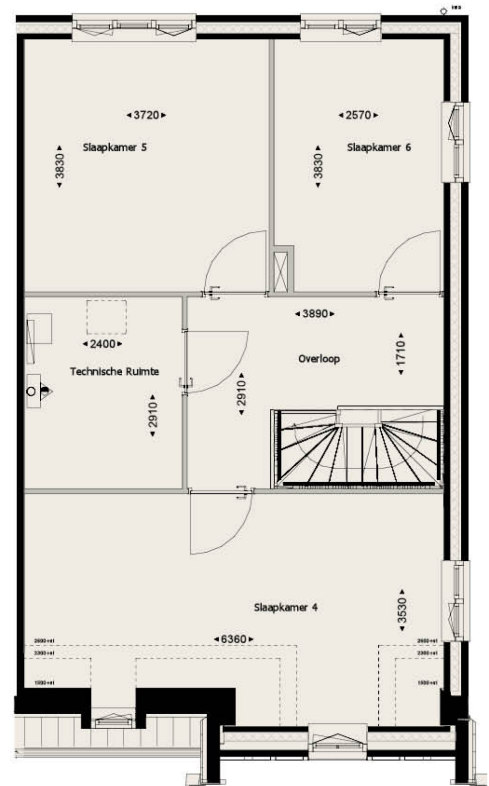
Tweede verdieping bouwnummer 40 en 42 (zoals afgebeeld) en 39, 41 en 43 (gespiegeld)
