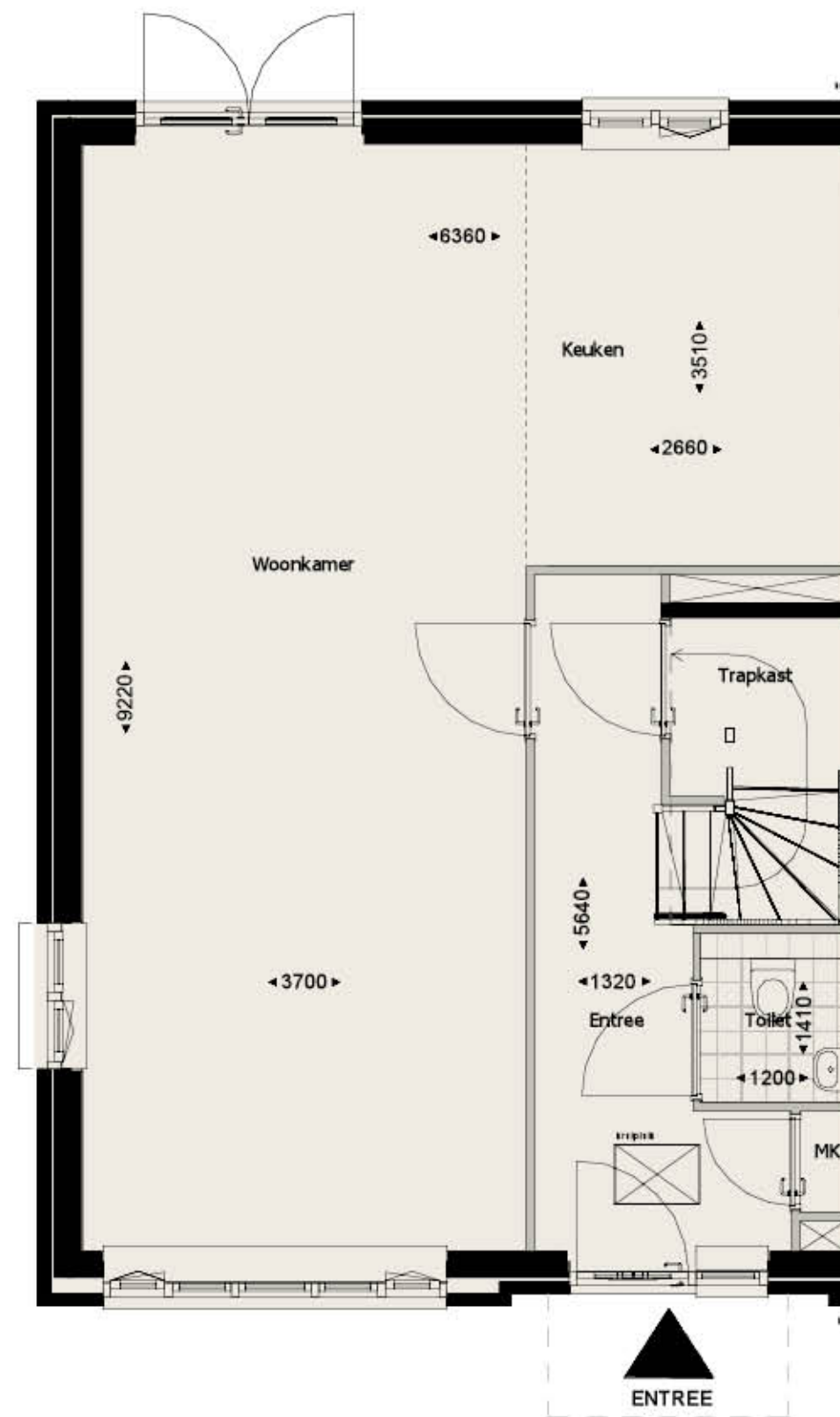
Begane grond bouwnummer 30 en 33 (zoals afgebeeld) en 31 en 27 (gespiegeld)
