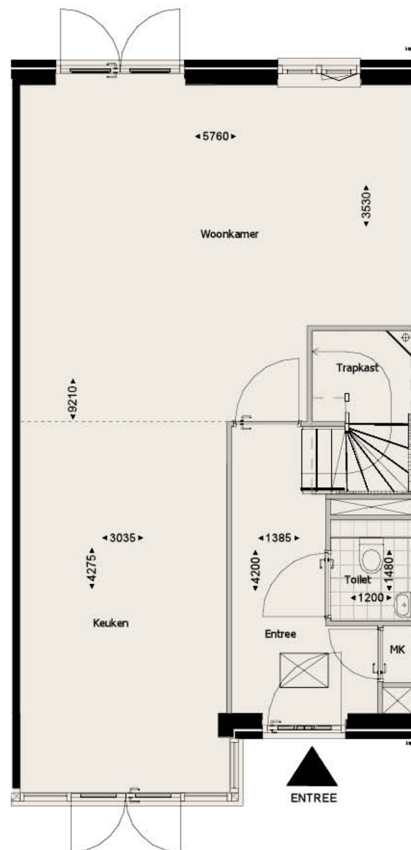
Begane grond bouwnummer 2 (zoals afgebeeld) en 3 (gespiegeld)
