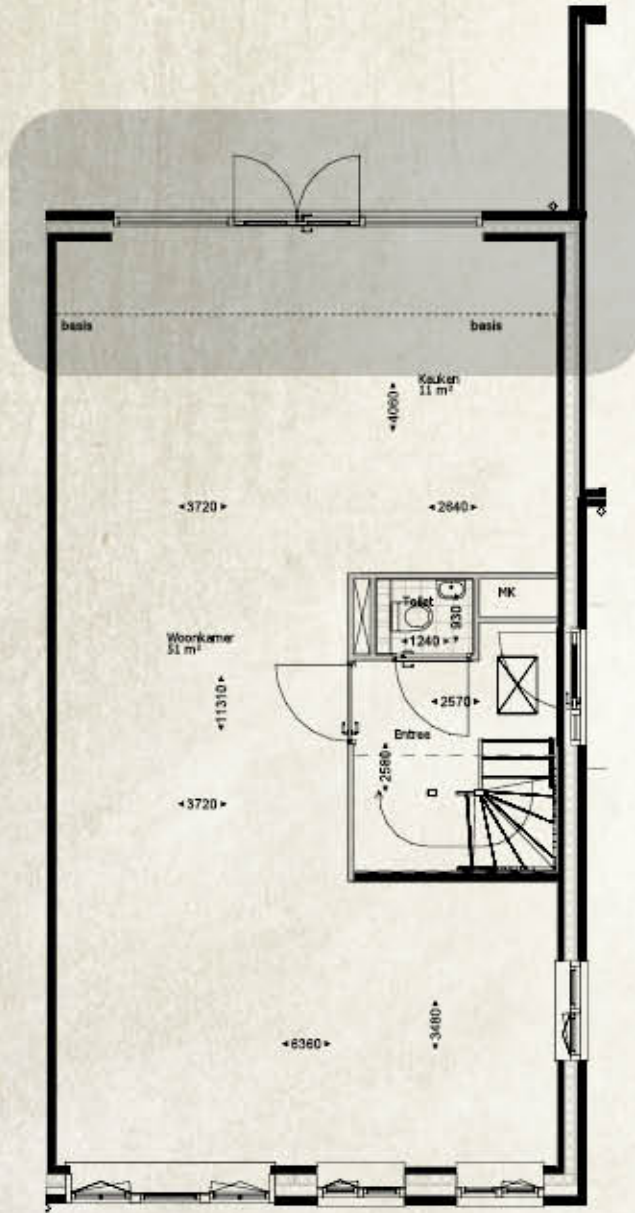
Uitbouw 0.9m Plattegrond op basis van Type D1
