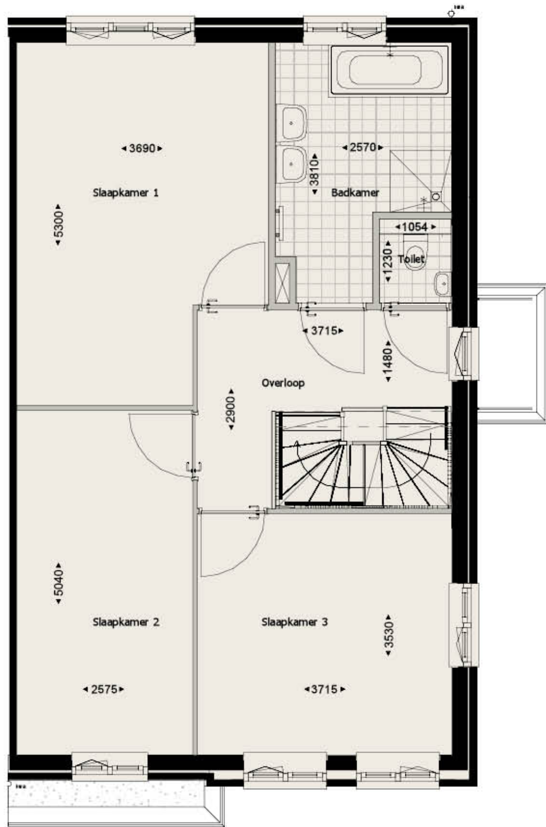
Eerste verdieping bouwnummer 38 (zoals afgebeeld)
