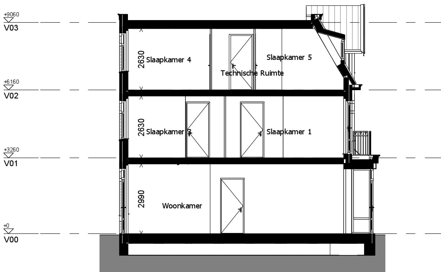
Doorsnede
