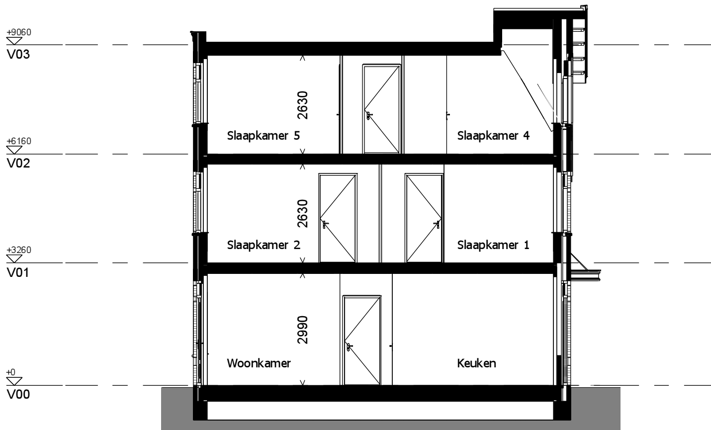
Doorsnede
