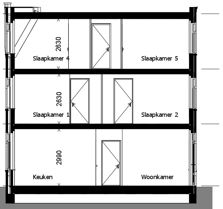
Doorsnede
