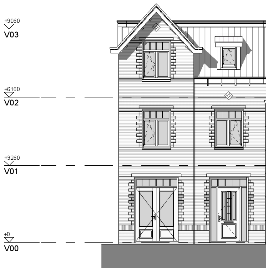
Voorgevel
