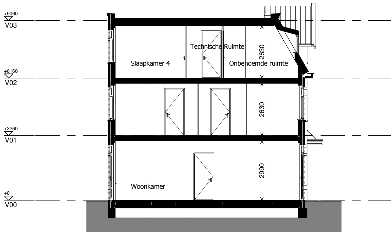
Doorsnede
