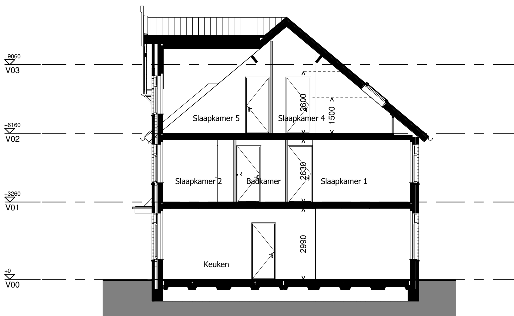
Doorsnede
