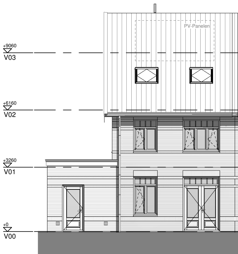
Achtergevel
