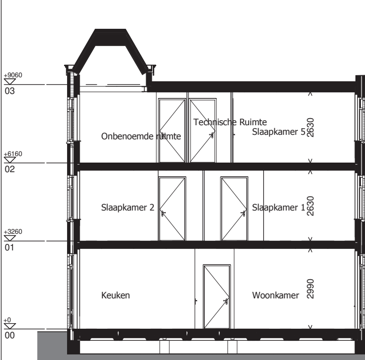
Doorsnede
