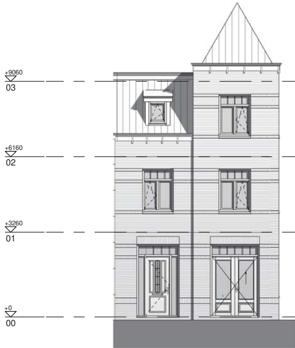
Vorgevel
