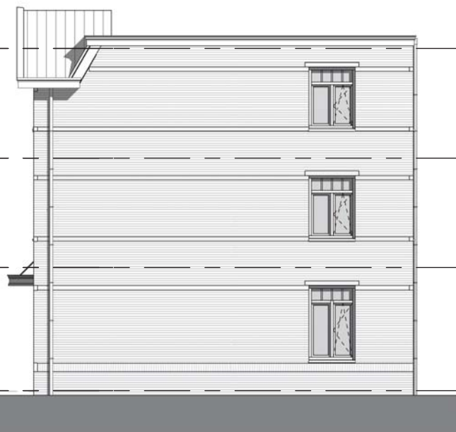
Zijgevel
