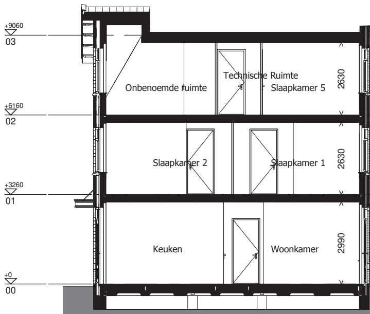
Doorsnede
